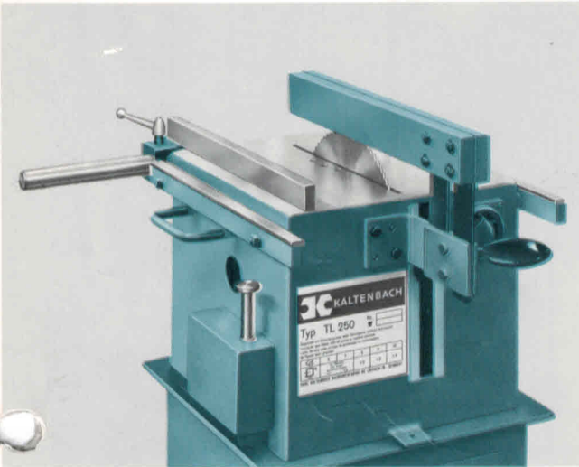
Längsschnittanschlag (Abb. 5)
