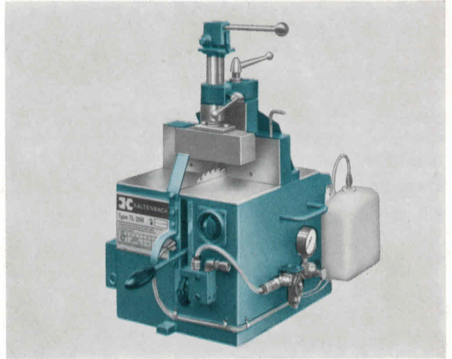
Kühlnebelsprühgerät (Abb. 4)
