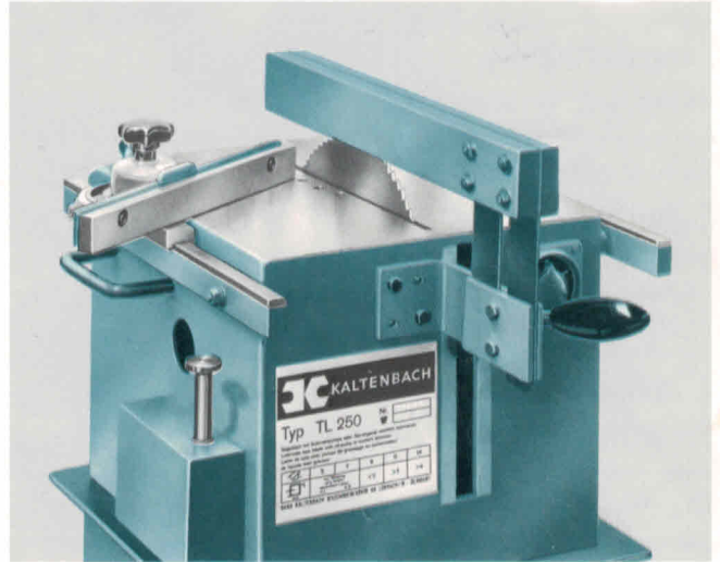
Schiebeanschlag (Abb. 6)
