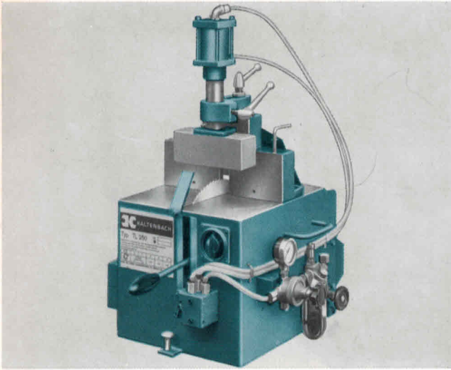
Preßluftspannstock (Abb. 3)
